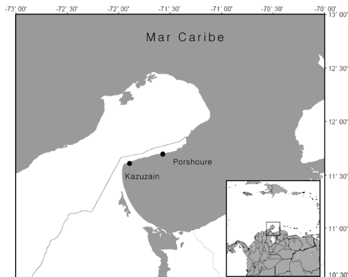
Figura 1. Mapa del área de estudio. Proyección Mercator. Tomado de MapTool ( www.seaturtle.org/maptool ).
